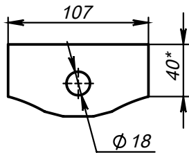
Поз.4 (Ушко) развёртка
